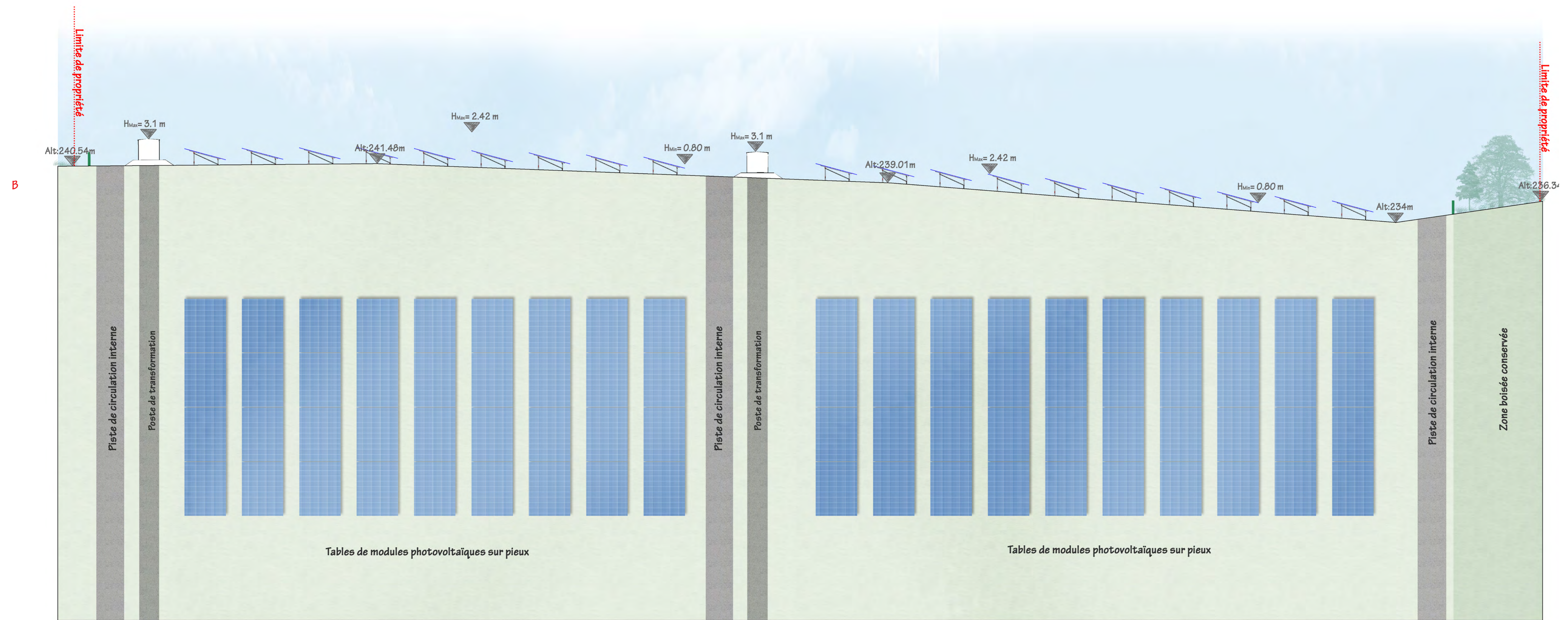
COUPE BB' : NORD/SUD DES PANNEAUX PHOTOVOLTAIQUES - échelle 1/300e
