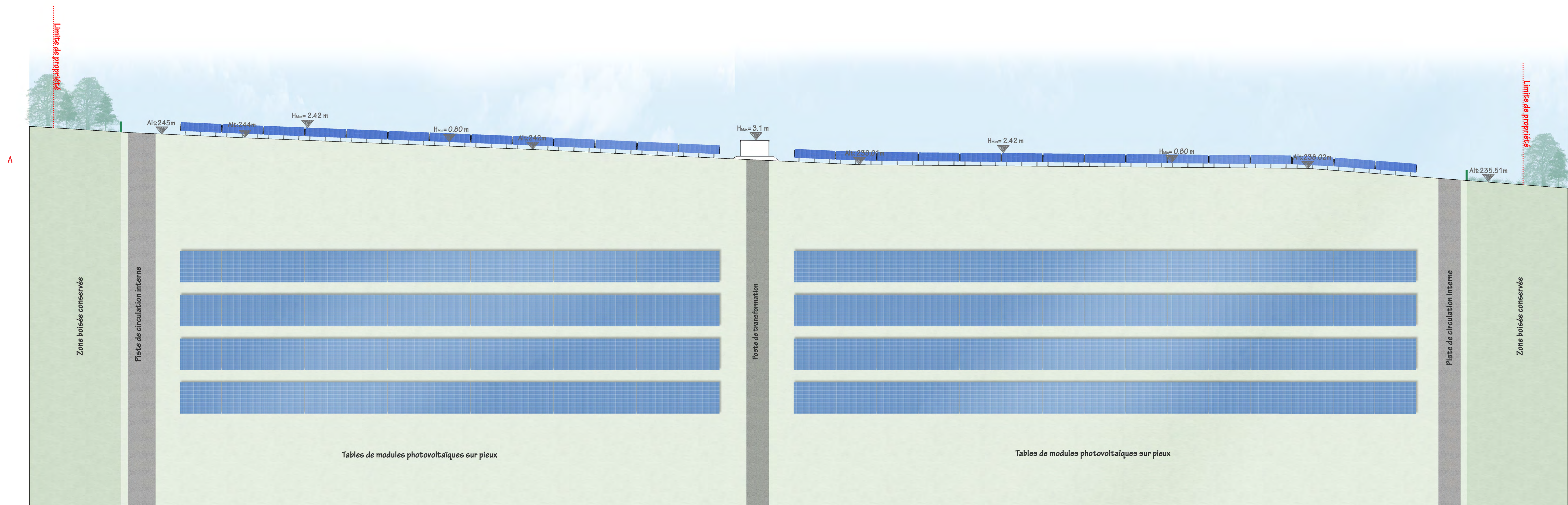
COUPE AA' : OUEST / EST DES PANNEAUX PHOTOVOLTAIQUES - échelle 1/300e
